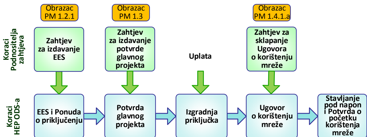
Slika 3. Prikaz koraka pri jednostavnom priključenju na distribucijsku mrežu ako u EES nije uvjetovan pokusni rad
