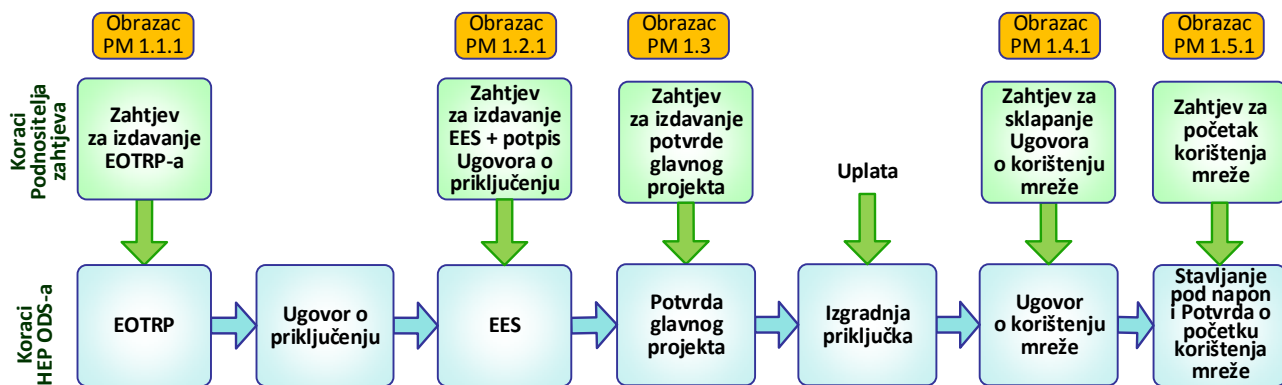
Slika 5. Prikaz koraka pri složenom priključenju na distribucijsku mrežu ako u EES nije uvjetovan pokusni rad
