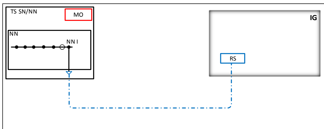
NN-I-4 Priključak u NN razvodu TS SN/NN (uvijek je jedan glavni vod korisnika mreže, koji po potrebi može biti izveden paralelnim kabelima, a počinje u jednoj točki u NN razvodu)
