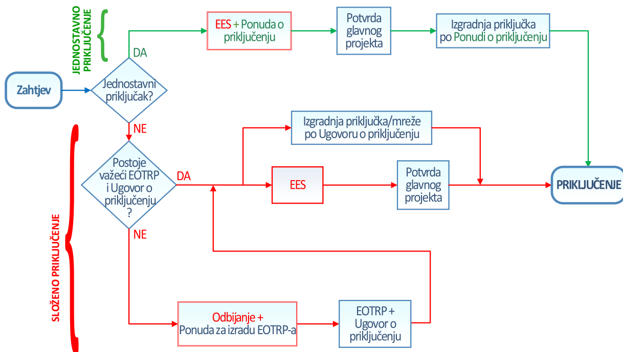
Slika 1. Vrste postupka priključenja
