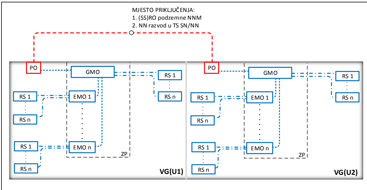
NN-V-2 Podzemni priključak u (SS)PO + GMO + EMO-i
