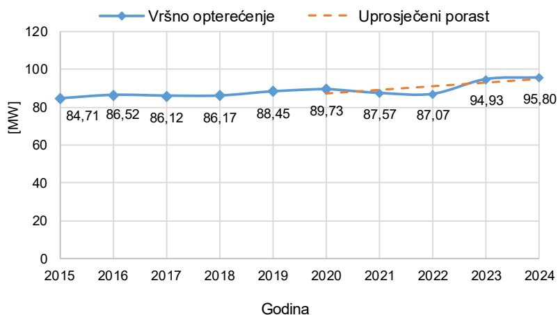
Ostvarena vršna opterećenja u razdoblju 2015. – 2024.
