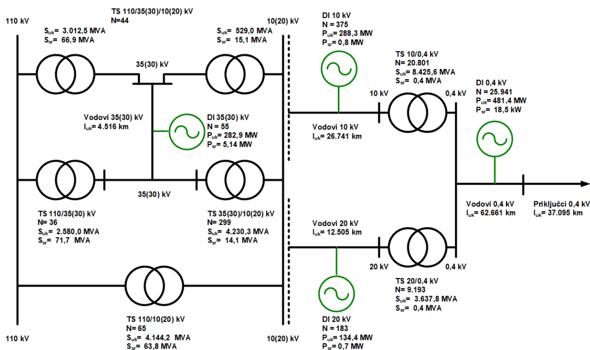
Slika 3-2 Pojednostavljeni rekapiulacijski shematski prikaz distribucijske mreže
