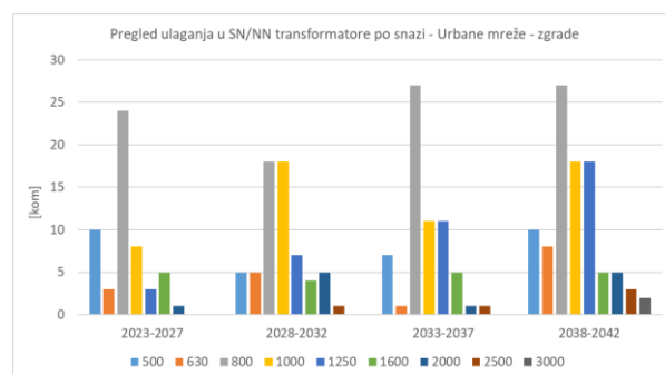
Slika 5-16 Broj potrebnih novih SN/NN transformatora za klaster Urbane mreže - zgrade
