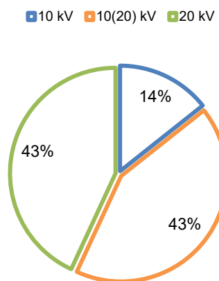
Slika 3-5 Trend promjene raspodjele polja SN postrojenja TS 110 kV prema pogonskom i konstrukcijskom naponu
