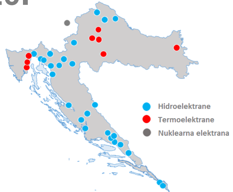
Proizvodnja električne energije u 2020
