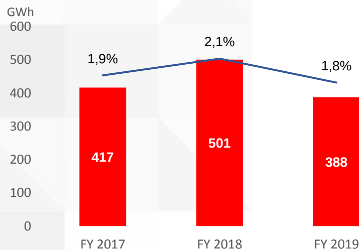
Gubici prijenosne mreže 1
