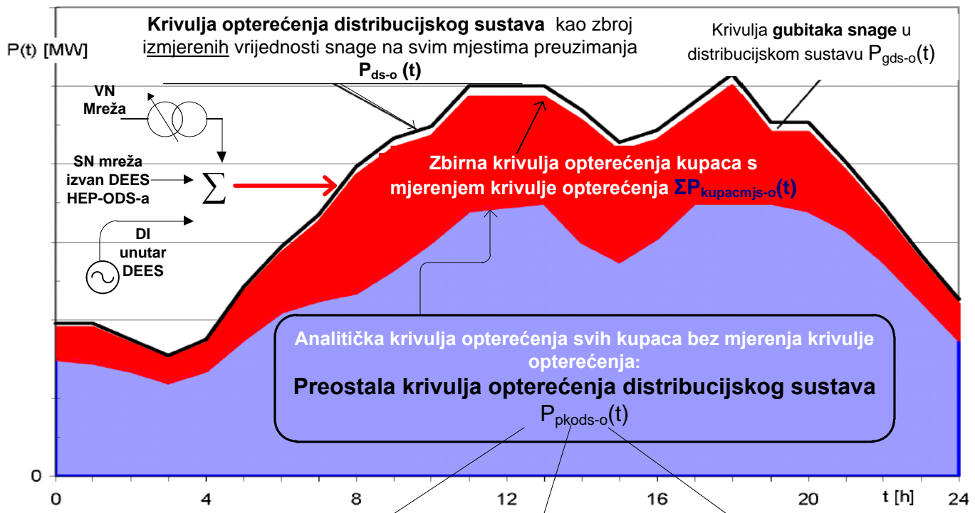
Krivulje ostvarenja KSK 1 do n
